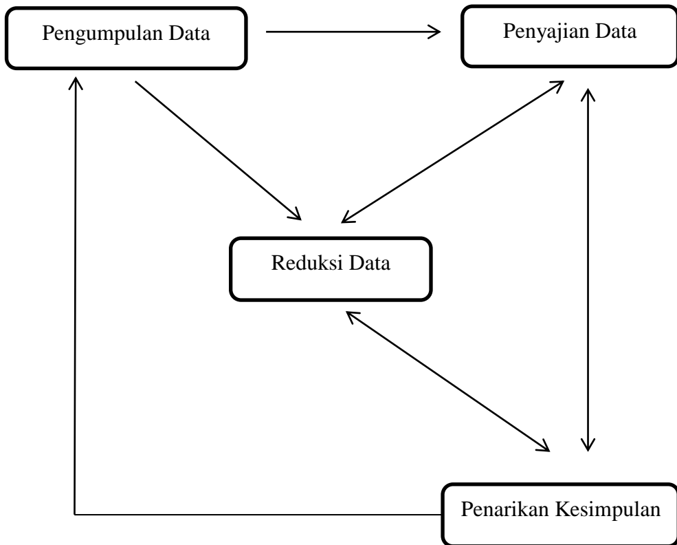
Gambar 3.1 Model Analisis Data Interaktif dari Miles dan Huberman.
